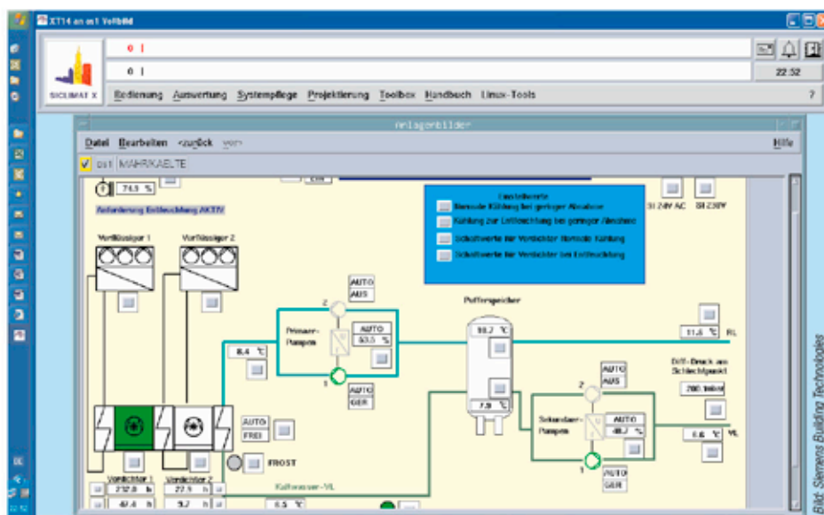
Anlagenbild Kälteerzeugung mit Primär- und Sekundärpumpen.
